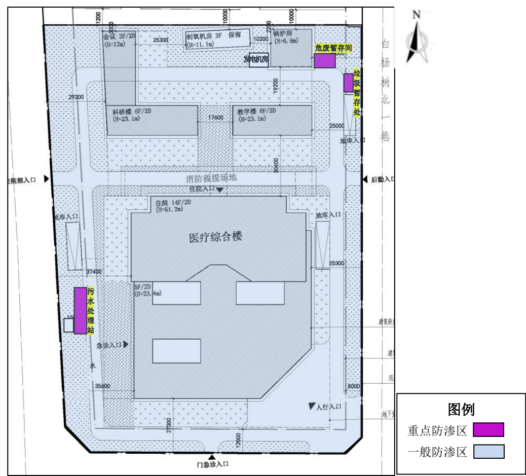
图 7.4-1 本项目分区防渗图
