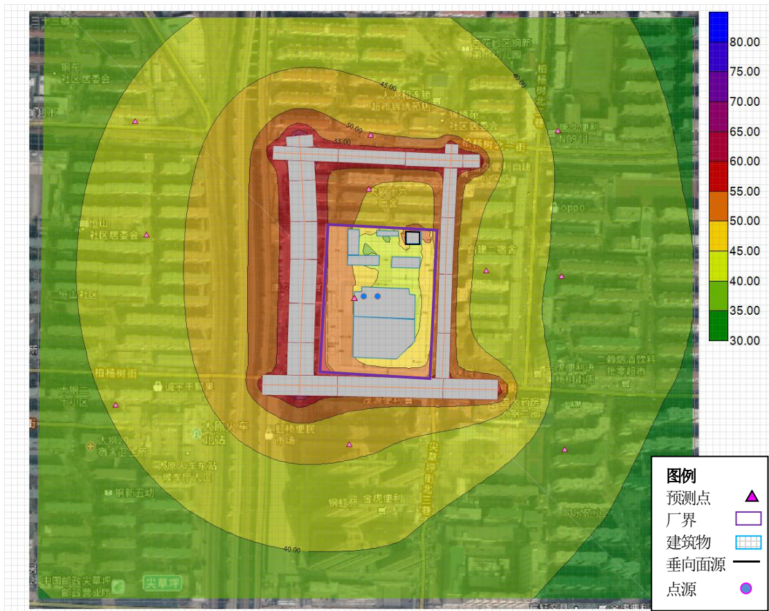
图 6.5-2 敏感点噪声预测等值线图
