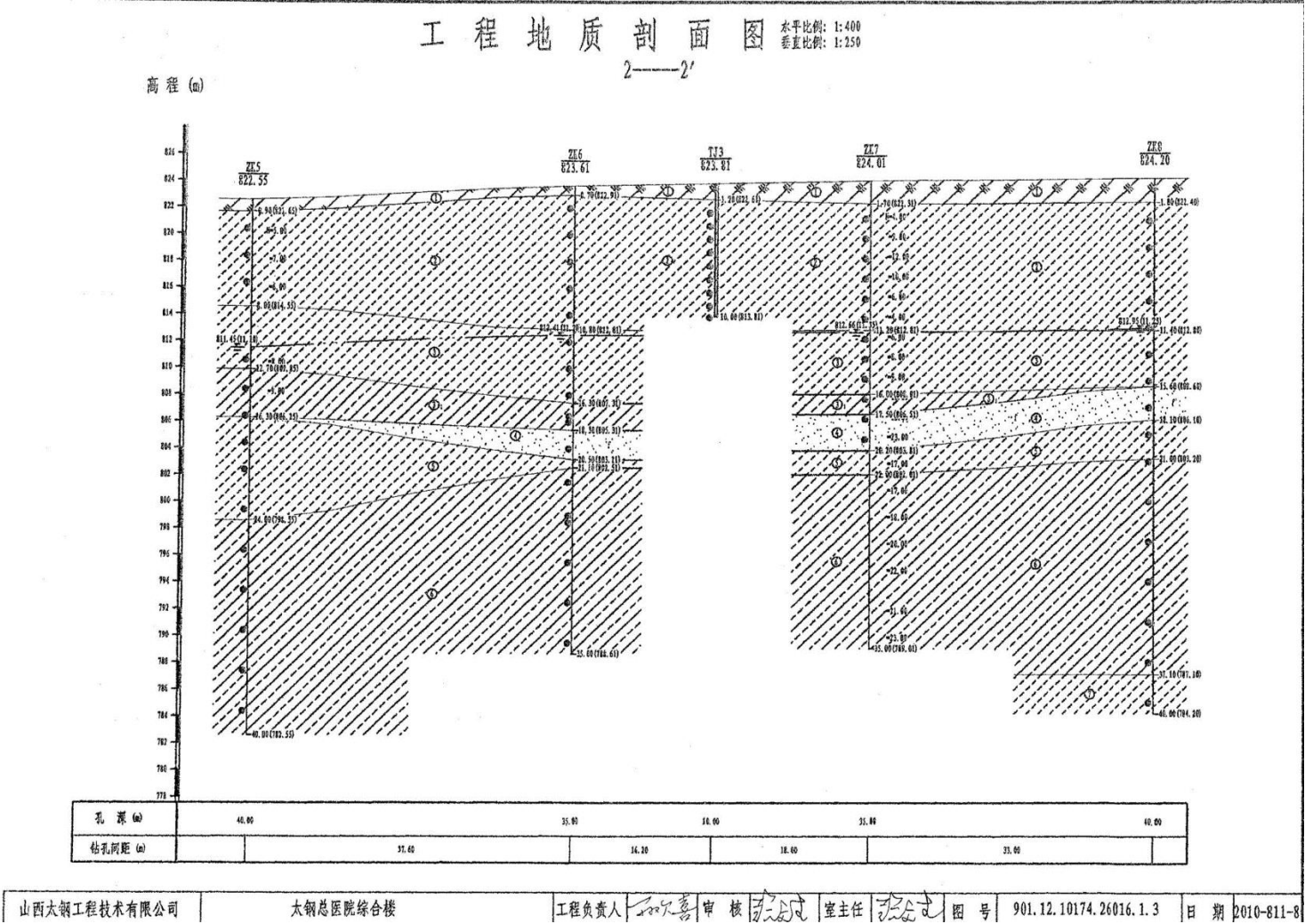
图 5.4-8 项目勘察区钻孔剖面图 (2-2')
