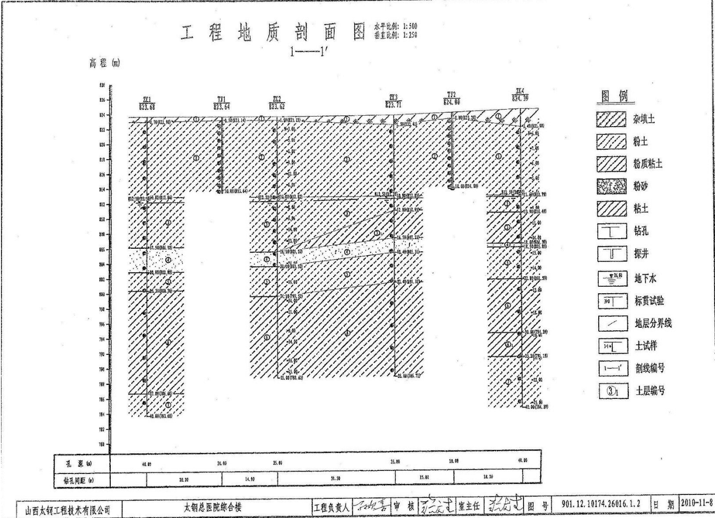
图 5.4-7 项目勘察区钻孔剖面图 (1-1')
